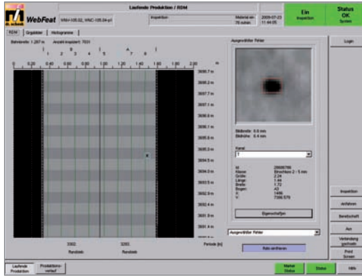
Die Running Defect Map gibt einen sofortigen Überblick über Fehler in der laufenden Produktion. Jeder Fehler ist als hochauflösendes Bild abrufbar.
