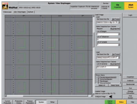
Gray Image Snapshot: Mikroskop-ähnliches Bild zur Kontrolle der Position von Sicherheitsmerkmalen.
